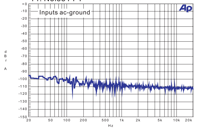
14. Noise FFT
